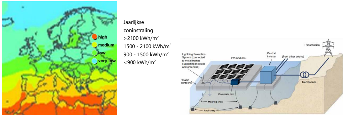
Afbeelding 4.5 Condities voor zonne-energie in Europa [60] (links) en onderdelen in een drijvend zonnepark [61] (rechts)
