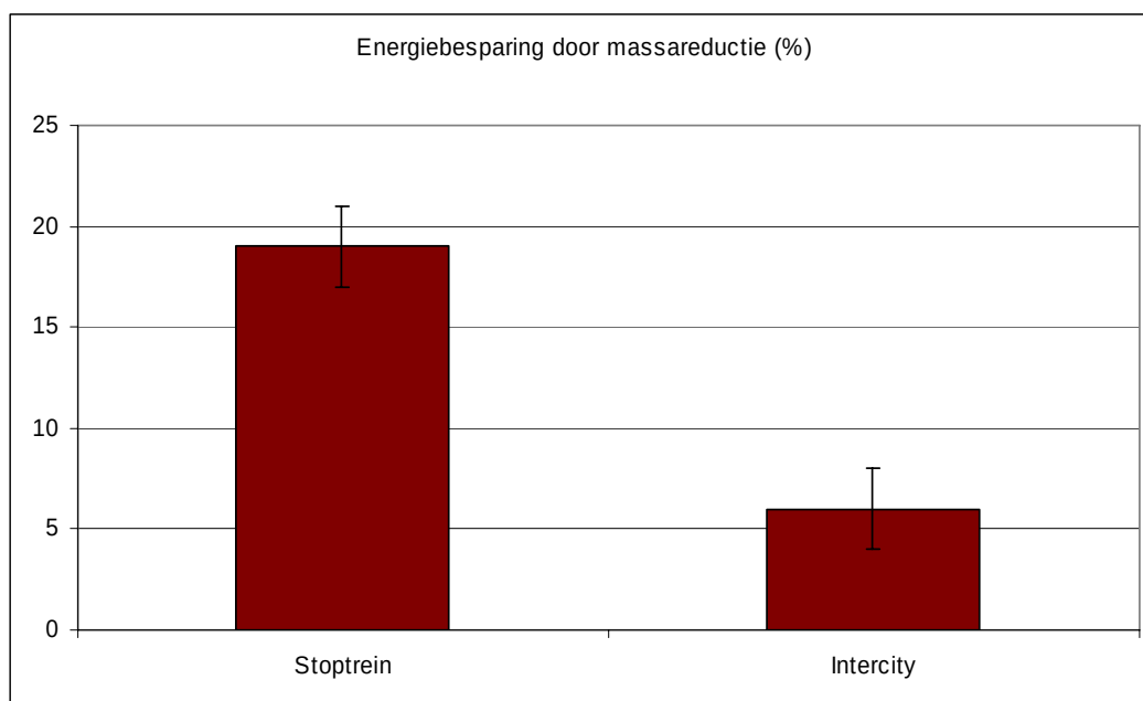
Figuur 19 Energiebesparing trein door massareductie
