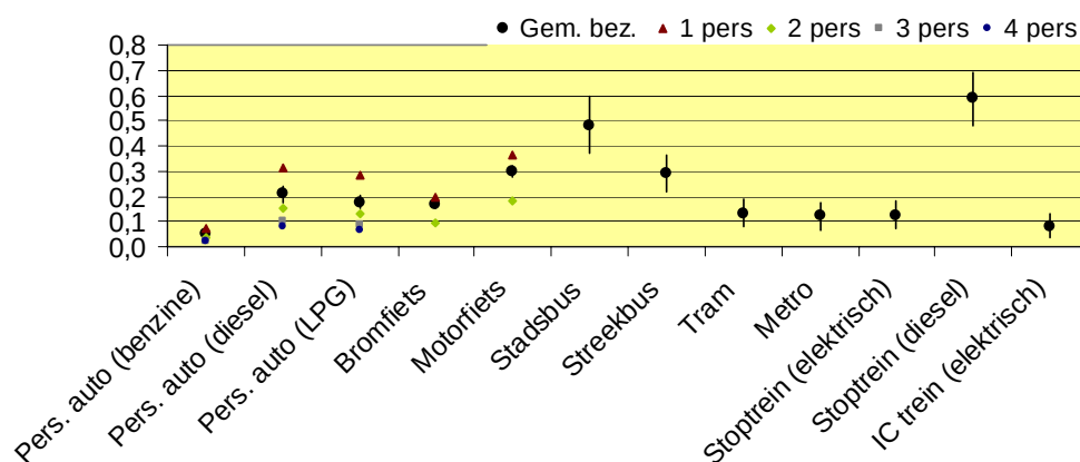
PM10 (g/rzg-km); korte afstand; dag gemiddelde; 2020
