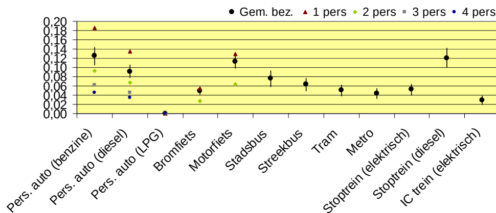
SO2 (g/rzg-km); korte afstand; dag gemiddelde; 2005
