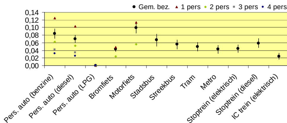
SO2 (g/rzg-km); korte afstand; dag gemiddelde; 2020
