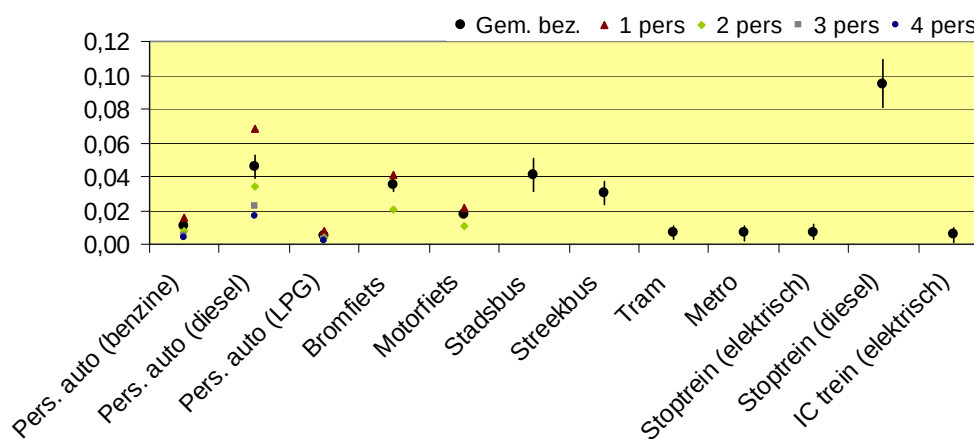
SO2 (g/rzg-km); korte afstand; dag gemiddelde; 2005
