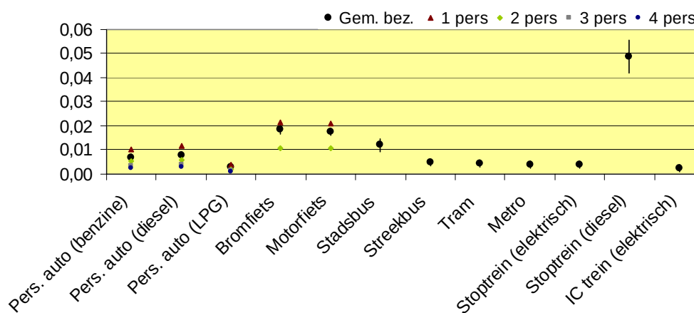
SO2 (g/rzg-km); korte afstand; dag gemiddelde; 2020
