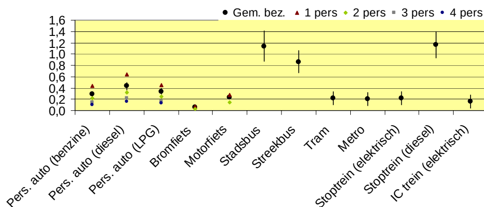
PM10 (g/rzg-km); korte afstand; dag gemiddelde; 2005
