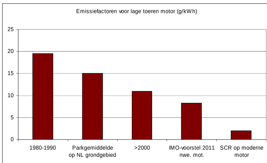
Figuur 26 Verskil in NO x -emissiefactoren in de zeescheepvaart
