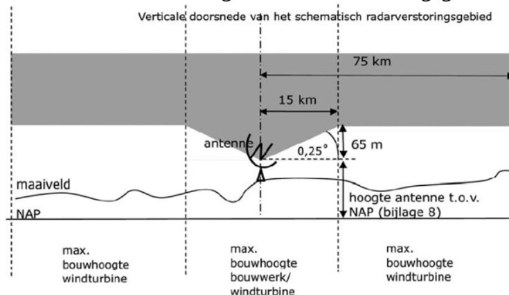
Schematische weergave bouwhoogte i.r.t. radarverstoring
