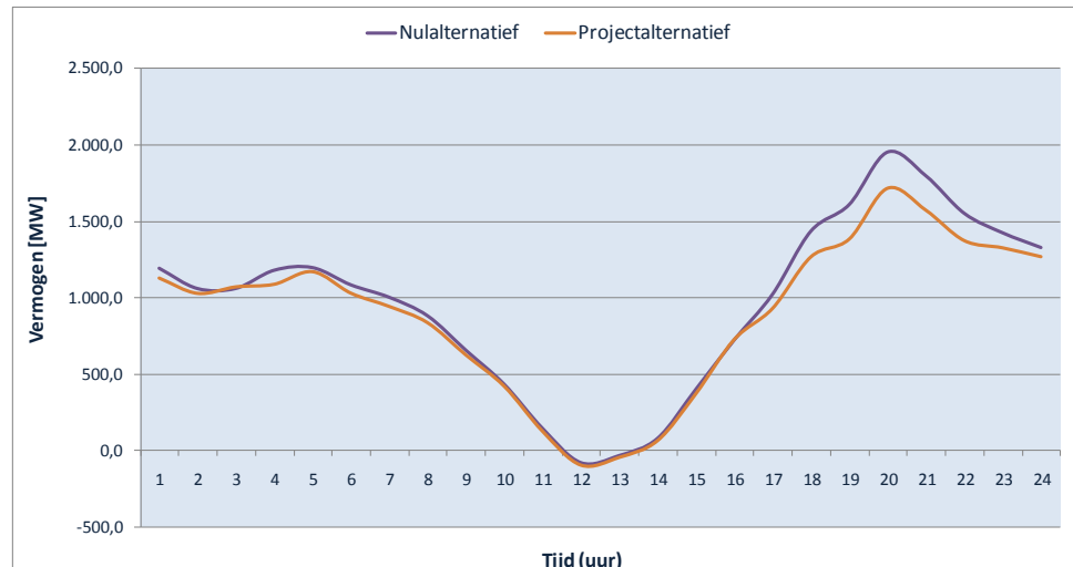
Figuur 23 Gemiddeld profiel voor de gebruikersgroep stedelijk bestaand in nul- en projectalternatief
