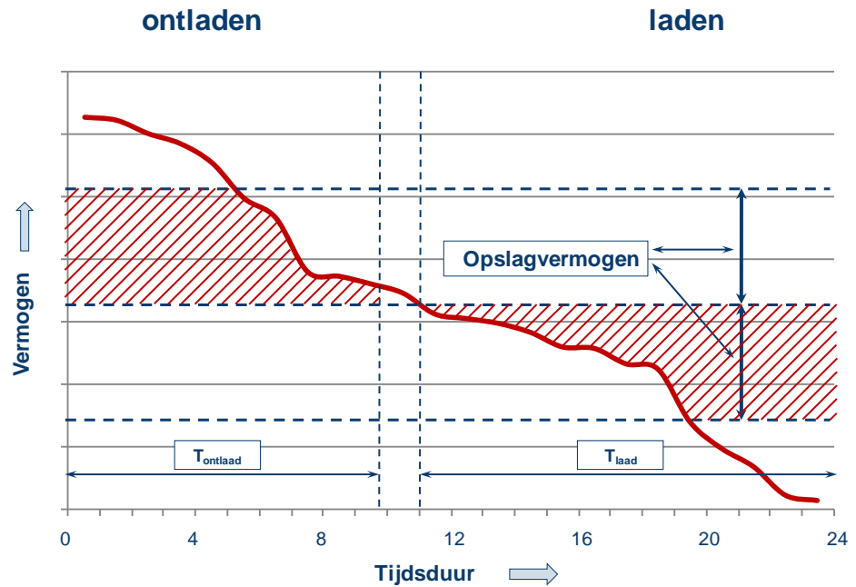
Figuur 36 Bepalen van tijdstippen van laden en ontladen op basis van een gesorteerde belastingkromme voor de netbelasting
