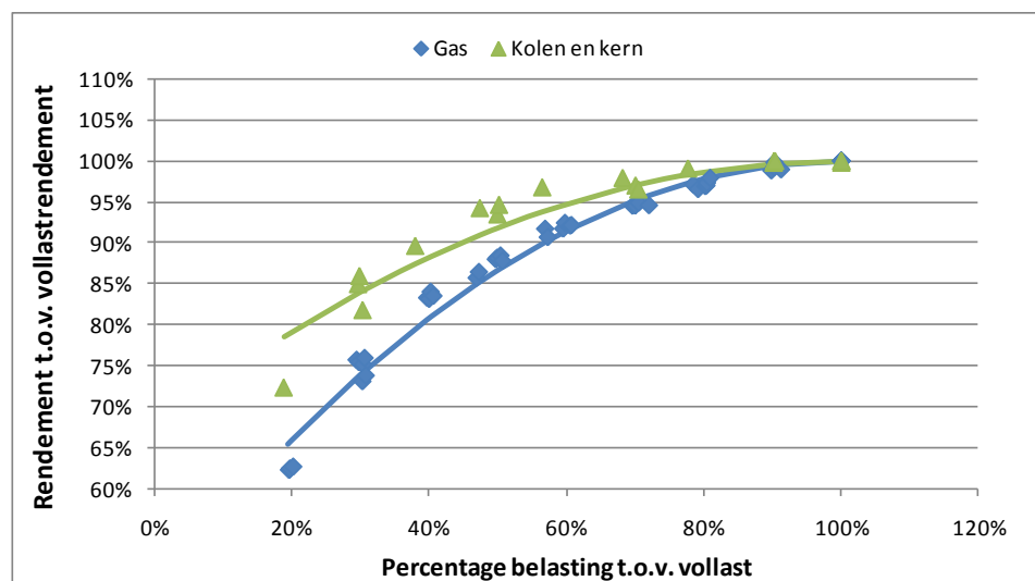
Figuur 44 Rendementsafname bij afname belastingpercentage voor centrale opwekeenheden
