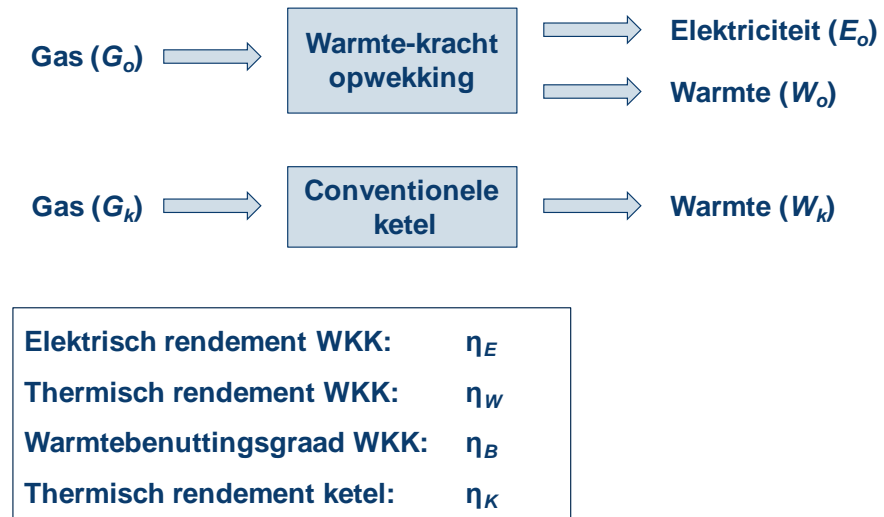
Figuur 43 Schematische weergave van voor berekening van de mark-up warmtelevering
