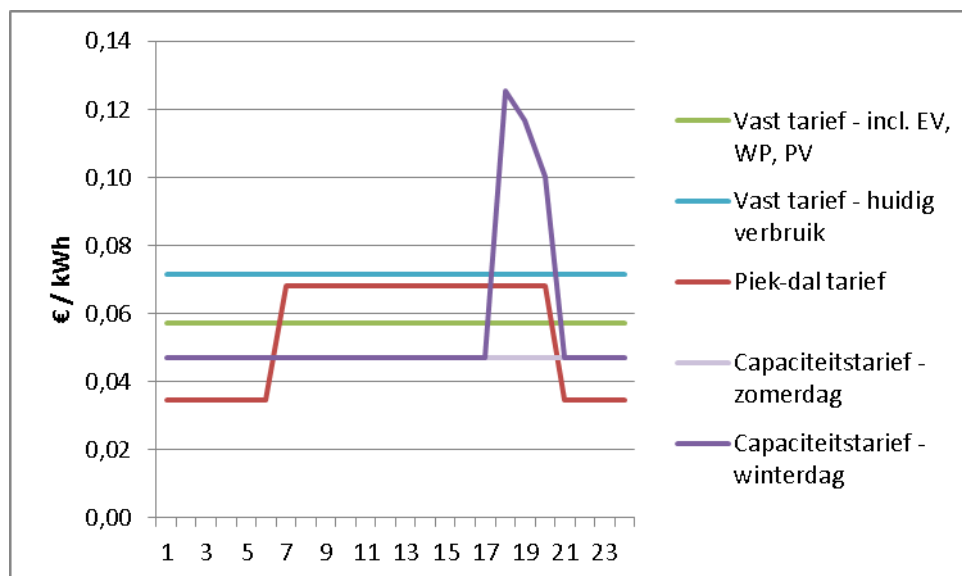
Figuur 20 Transportkosten per kWh in de verschillende tariefschema's
