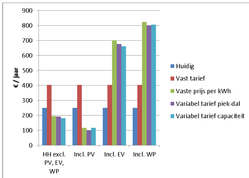
Figuur 24 Transporttarief van vier verschillende huishoudens
