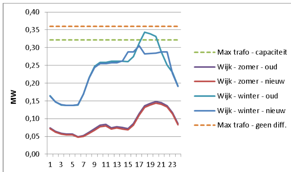
Figuur 19 Wijkprofielen met variabele tarieven op basis van capaciteit
