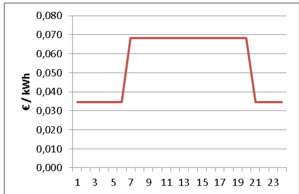
Figuur 16 Transporttarief dal en piek
