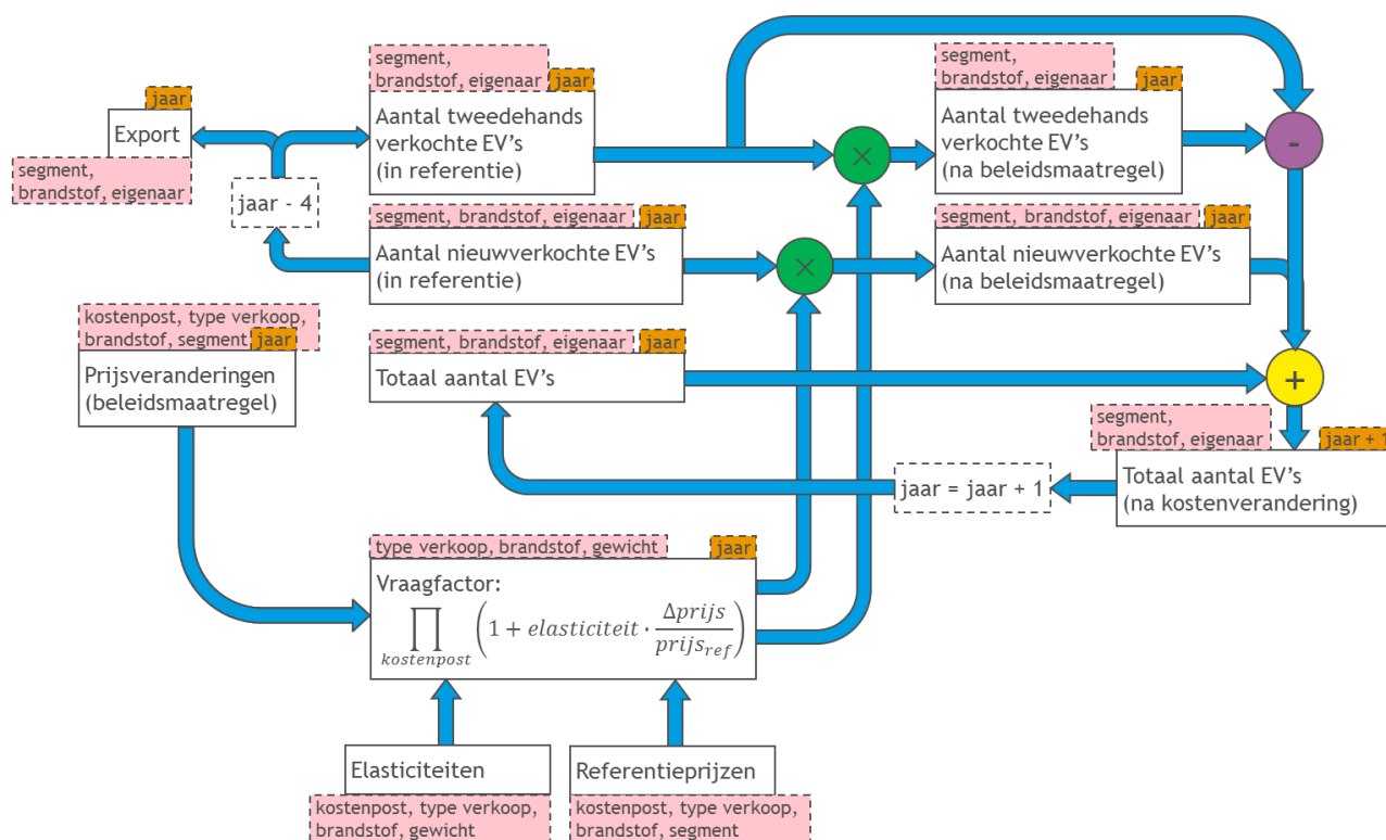
Figuur 7 Overzichtsschema gegevensstromen CEPAIA
