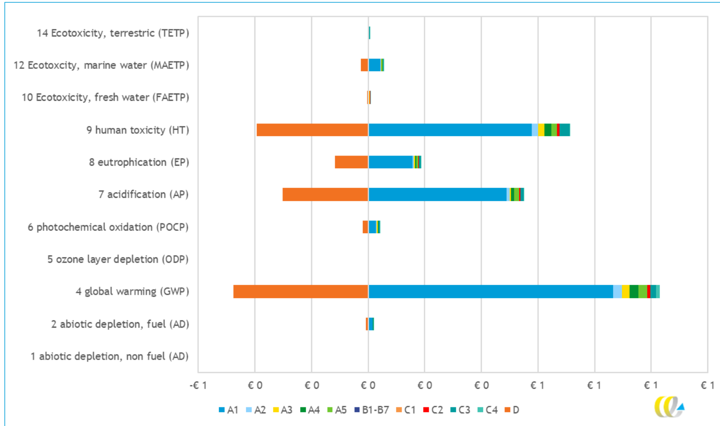
Figuur 6 - Gewogen milieuprofiel (MKI, in €) van één hardhouten paal van een meter, opgedeeld in levensfasen
