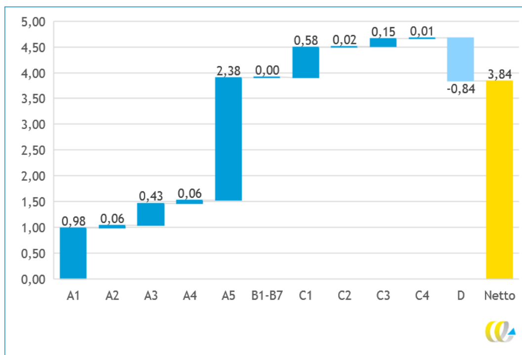
Figuur 3 - MKI-scores voor één vierkante meter beschoeiingselement van naaldhout en tropisch hardhout (exclusief palen)
