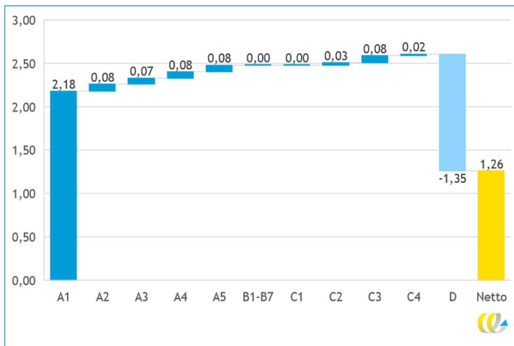
Figuur 4 - MKI-scores voor één stuk hardhouten paal van één meter
