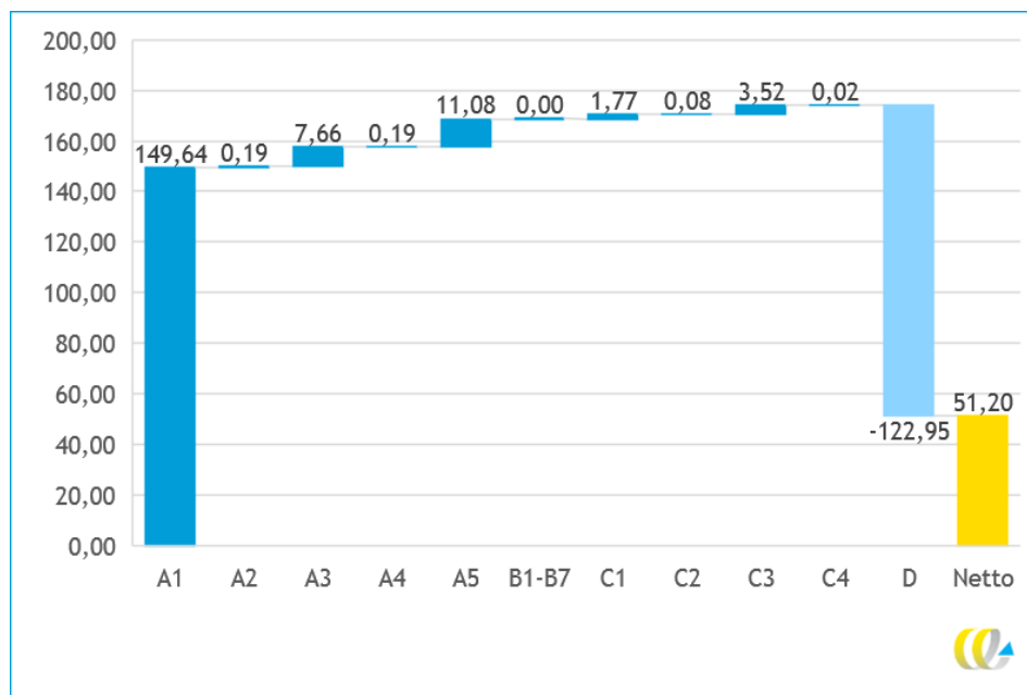
Figuur 5 - MKI-scores voor één vierkante meter damwand van Europees naaldhout en gerecycled kunststof, opgedeeld in levensfasen (exclusief 30% categorie-opslag)
