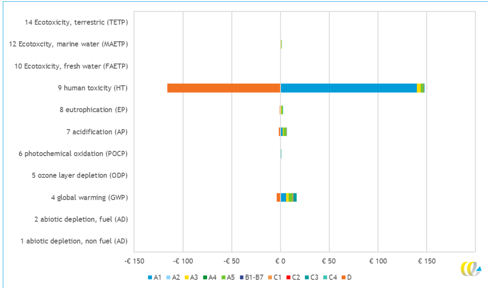
Figuur 6 - Gewogen milieuprofiel (MKI, in €) van één vierkante meter damwand van Europees naaldhout en gerecycled kunststof, opgedeeld in levensfasen (exclusief 30% categorie-opslag)
