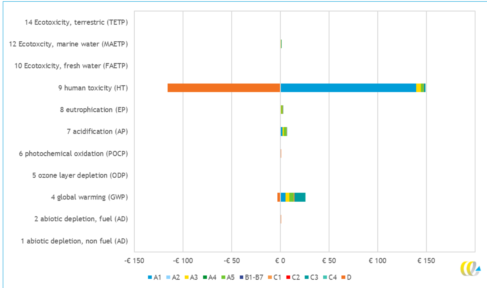
Figuur 5 - Gewogen milieuprofiel (MKI, in €) van één vierkante meter damwand van gerecycled kunststof, opgedeeld in levensfasen (exclusief 30% categorie-opslag)
