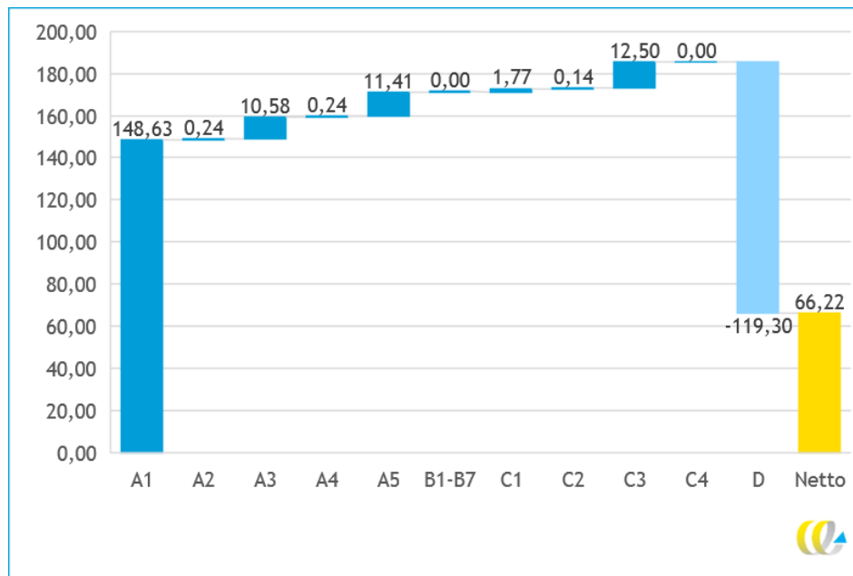
Figuur 4 - MKI-scores voor één vierkante meter damwand van gerecycled kunststof, opgedeeld in levensfasen (exclusief 30% categorie-opslag)
