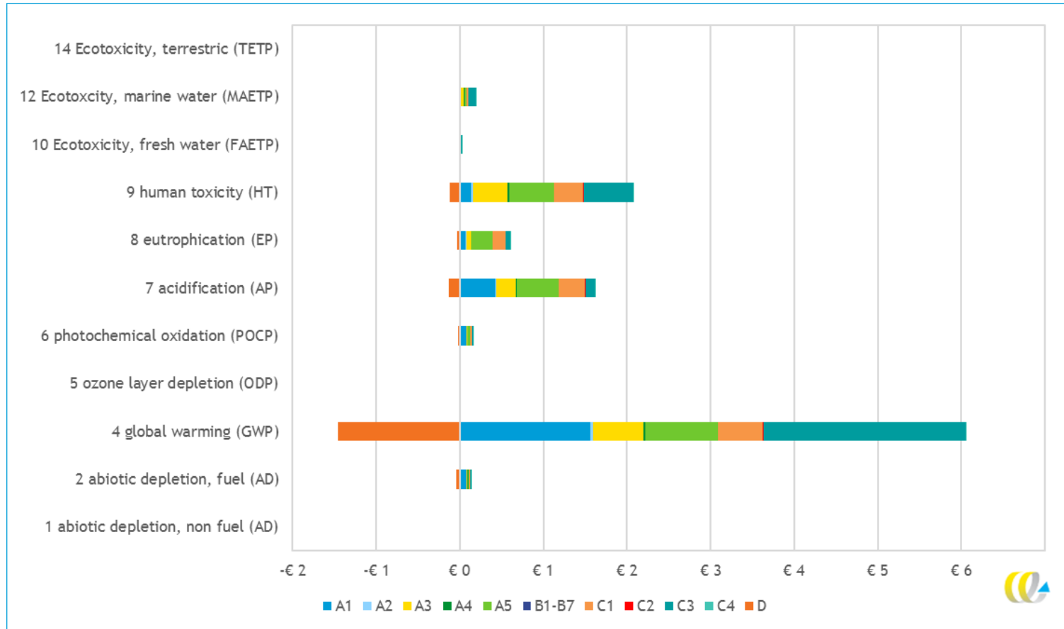
Figuur 4 - Gewogen milieuprofiel (MKI, in €) van één stuk duiker van PE, opgedeeld in levensfasen (exclusief 30% categorie-opslag)
