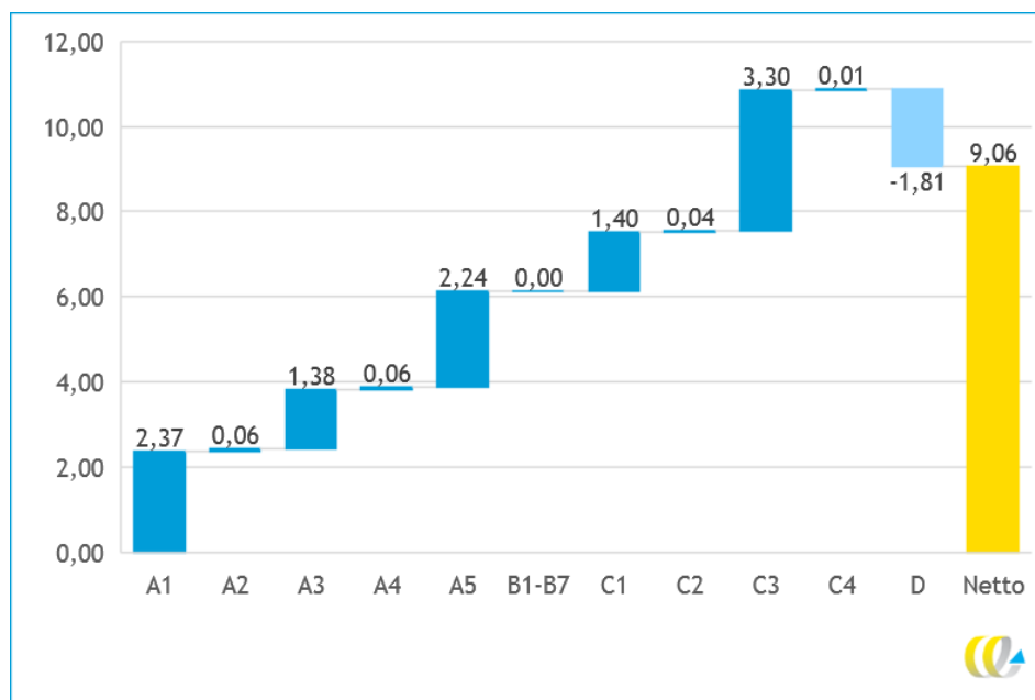
Figuur 3 - MKI-scores voor één stuk duiker van PE, opgedeeld in levensfasen (exclusief 30% categorie-opslag)
