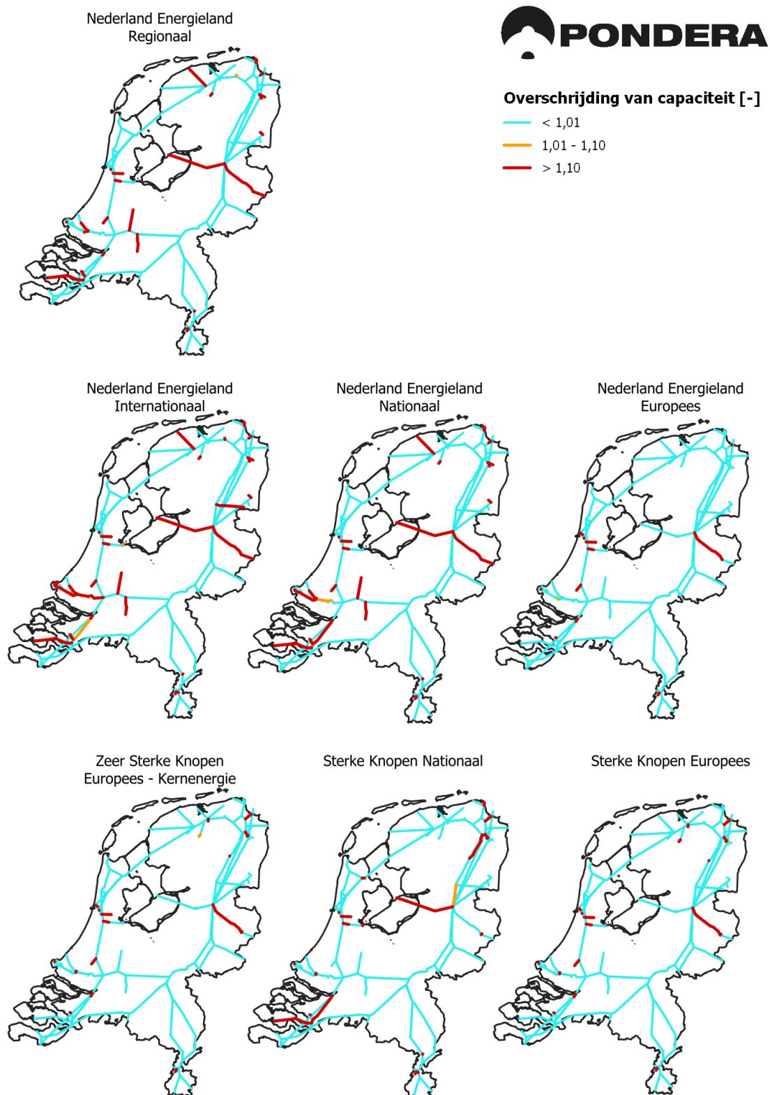
Figuur 3.1 - Resultaten doorrekening waterstofknelpunten in het HTL
