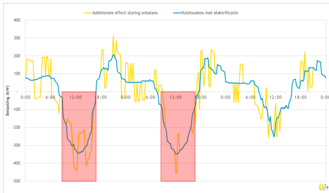
Figuur 2 - Voorbeeld visualisatie: Belasting van MSR met inzet van 10% thuisbatterij meeregelen op passieve onbalans (gele lijn) en zonder (blauwe lijn) gedurende 3 dagen in mei 2023. De rode blokken zijn uren met mogelijke beperking om hogere piekbelasting te voorkomen
