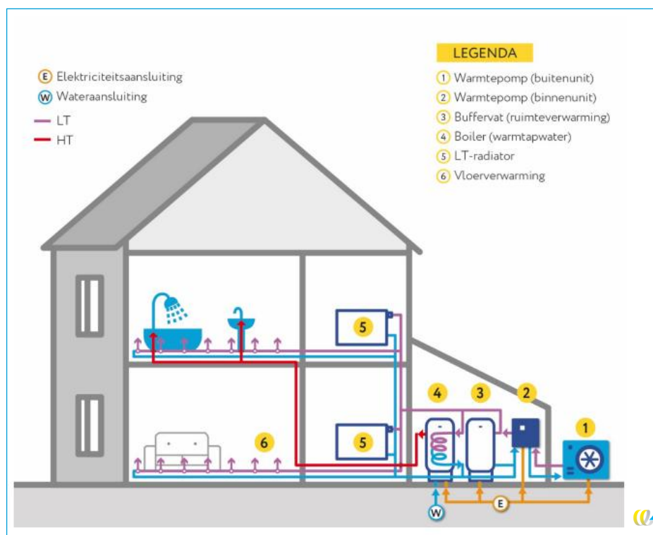
Figuur 8 - Schematische weergave lucht-waterwarmtepomp in een woning
