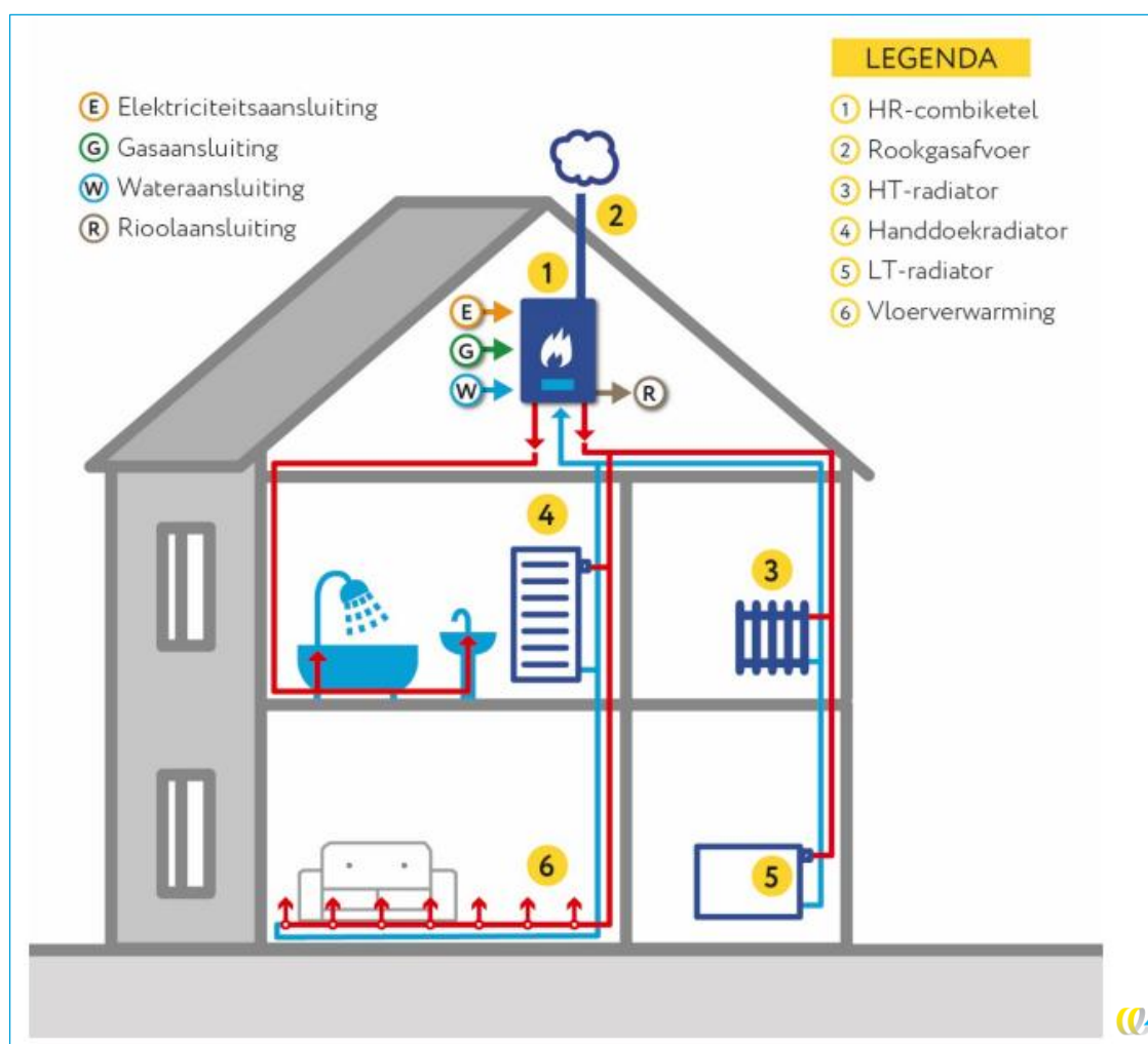
Figuur 9 - Schematische weergave hr-ketel
