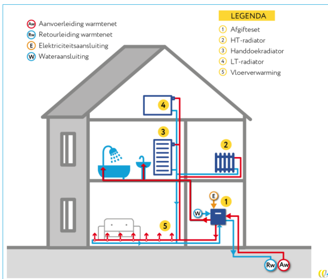
Figuur 12 - Schematische weergave mt-net
