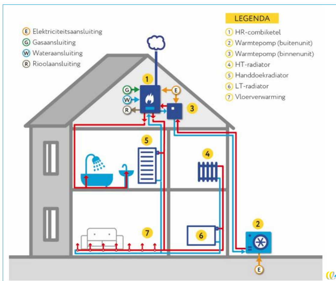
Figuur 10 - Schematische weergave hybride warmtepomp in een woning
