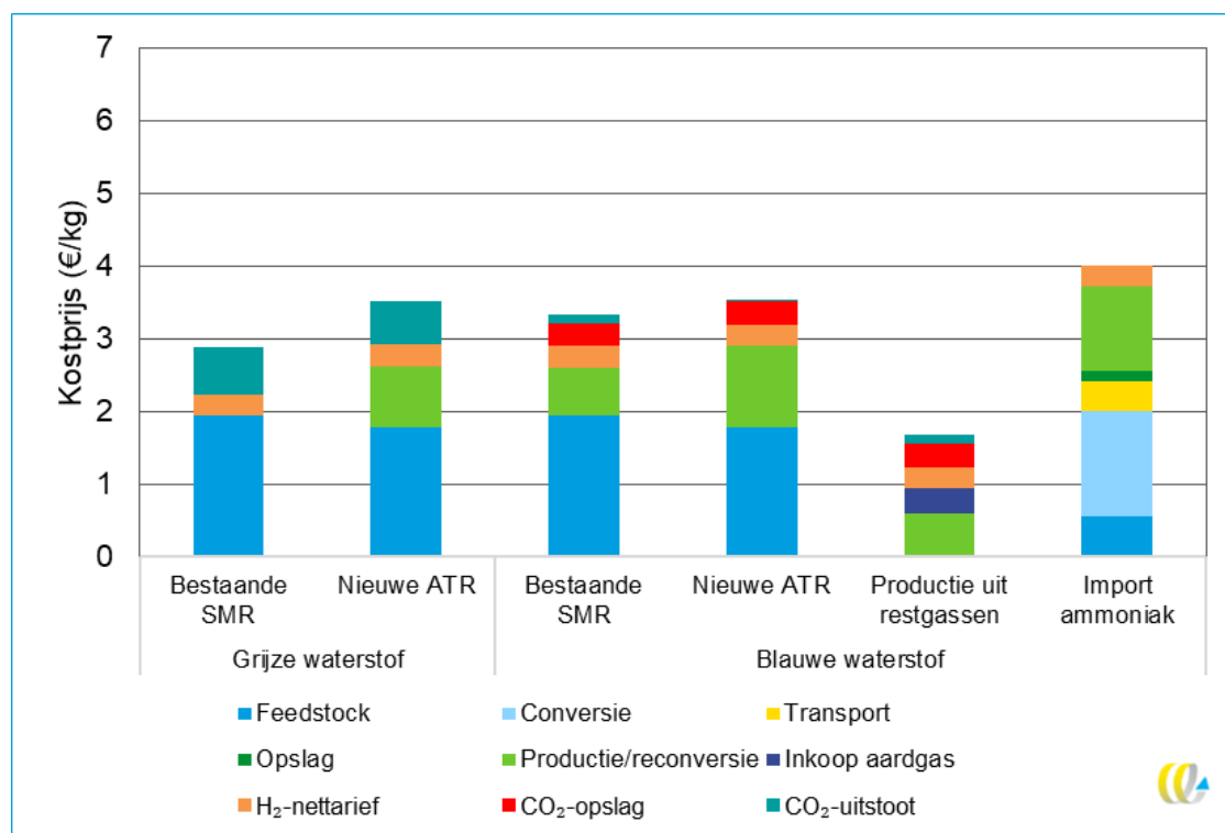
Figuur 5 – Kostprijzen productieroutes van grijze en blauwe waterstof in 2025, scenario Gemiddeld
